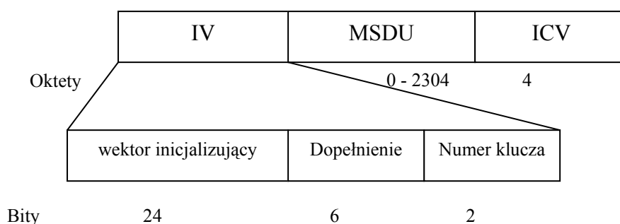
Rys.8. Ramka danych WEP
