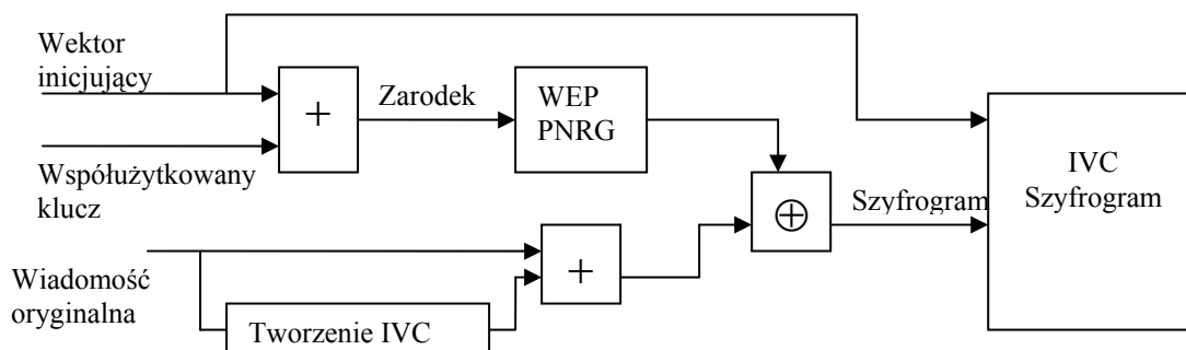
Rys.7. Mechanizm szyfrowania WEP
